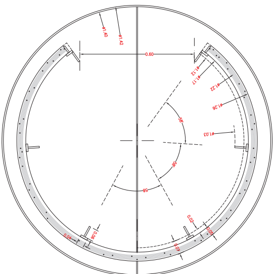
PLANTA COTES
