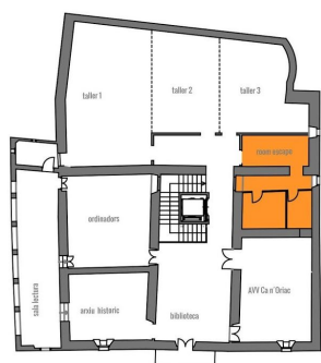
PLANTA PIS
